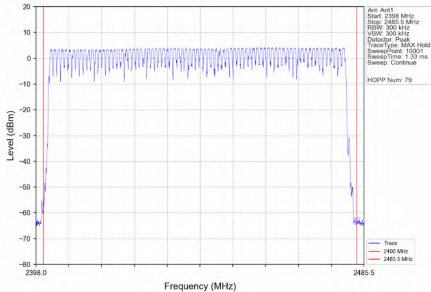
8DPSK_3DH5_HOPP_Ant1_NTNV
