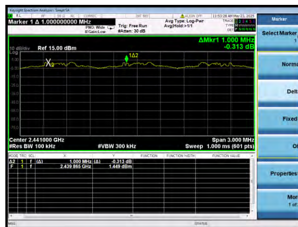
\pi/4 -DQPSK
