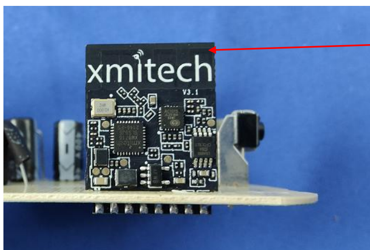
Antenna
