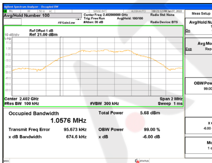
6dB BandwidthMode1 CH00
