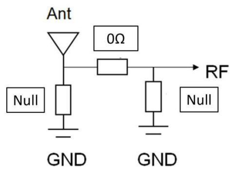
图 3 匹配电路
