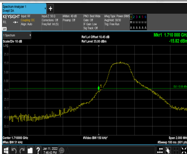
Band4-3MHz-QPSK-19965-1RB#14
