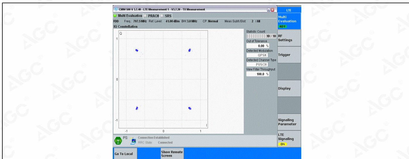
Band12-3MHz-QPSK-23165-15RB#0
