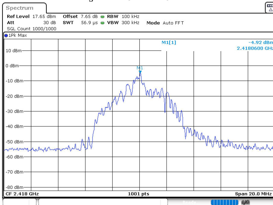
Band Edge NVNT GFSK 2418MHz Ant1 Ref
