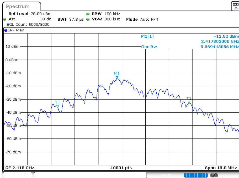
OBW NVNT GFSK 2418MHz Ant1
