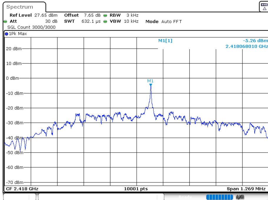
PSD NVNT GFSK 2418MHz Ant1
