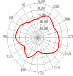
2500.000MHz E2
