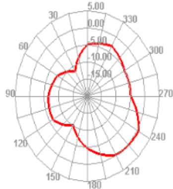
5150.000MHz E1
