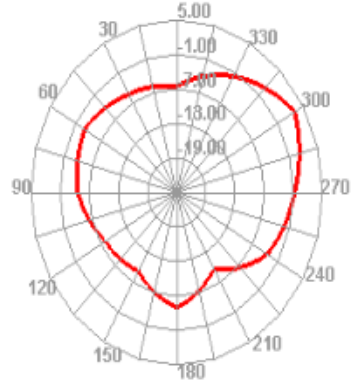
5150.000MHz H
