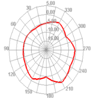
5150.000MHz E2
