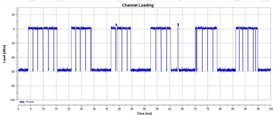
11AC80SISO_5610_Type0
