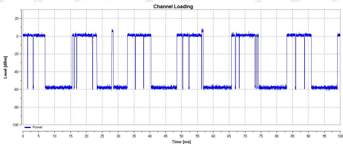
11AC80SISO_5610_Type0
