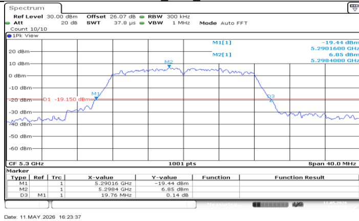
11A_Ant1_5300
