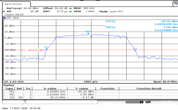
11A_Ant1_5620
