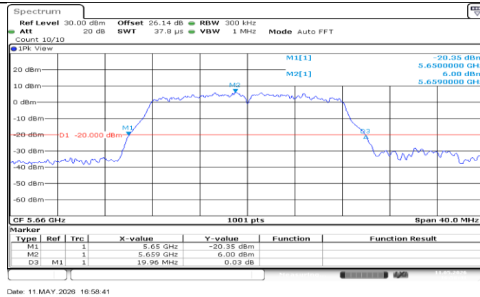
11A_Ant1_5660
