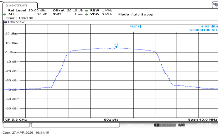
11A_Ant1_5300
