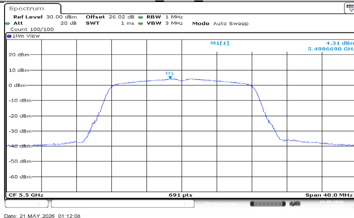
11A_Ant1_5500
