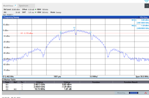
802.11b / 2 462 MHz
