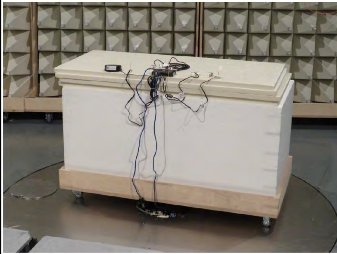
TEST SETUP: 1000-2000MHZ
