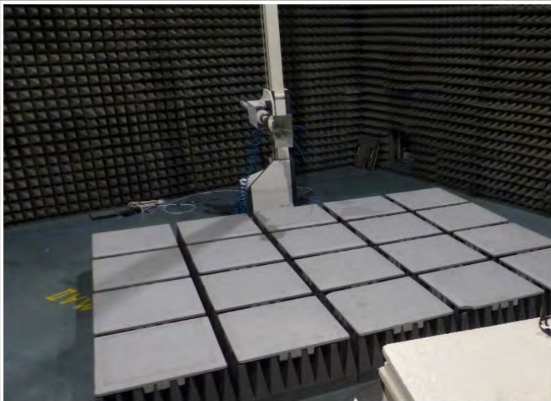
TEST SETUP: 1000-2000MHZ
