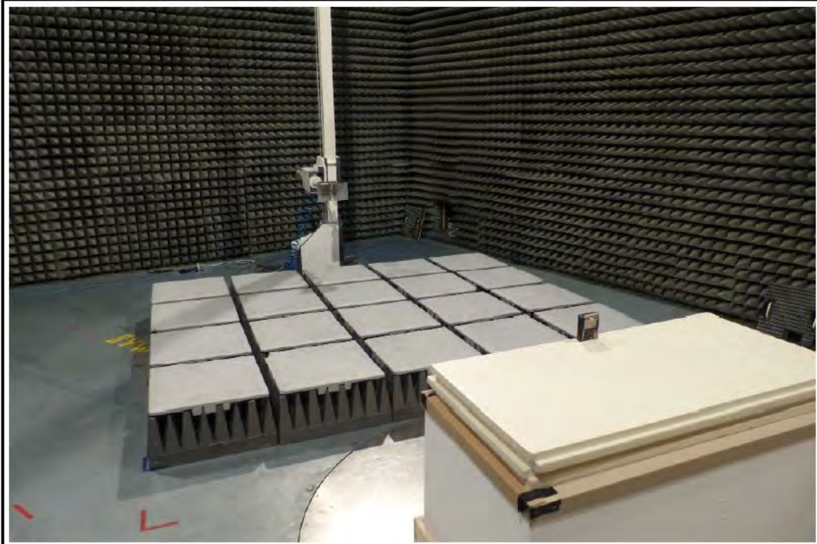
Test Setup 1000-13000MHz
