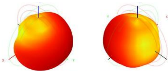
433.0MHz Total( E2-YZ), Max=- 2.13dBi
