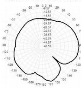
433.0MHz Total( E2-YZ), Max=- 2.13dBi
