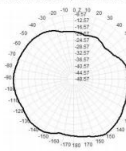
433.0MHz Total( E1-XZ), Max=- 2.45dBi
