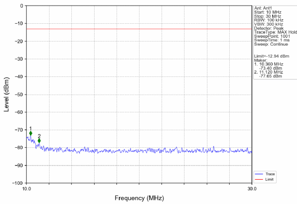
10MHz-30MHz
