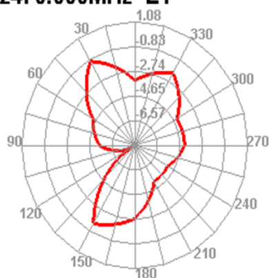
2470.000MHz E1
