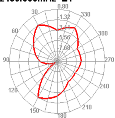
2480.000MHz E1
