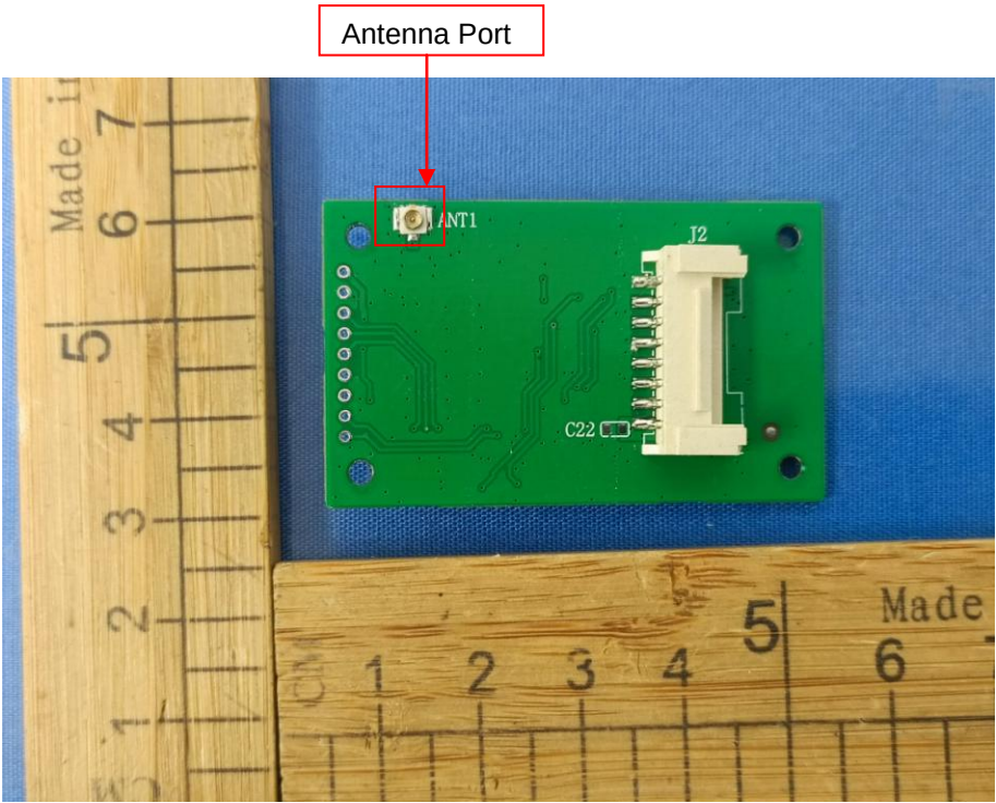
Antenna
