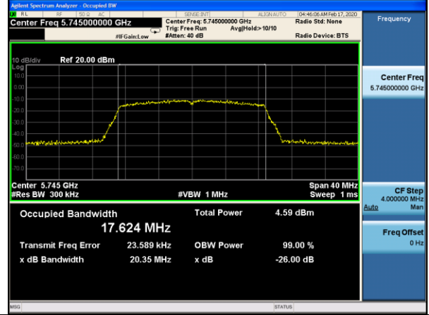
11n(HT20) CH149
