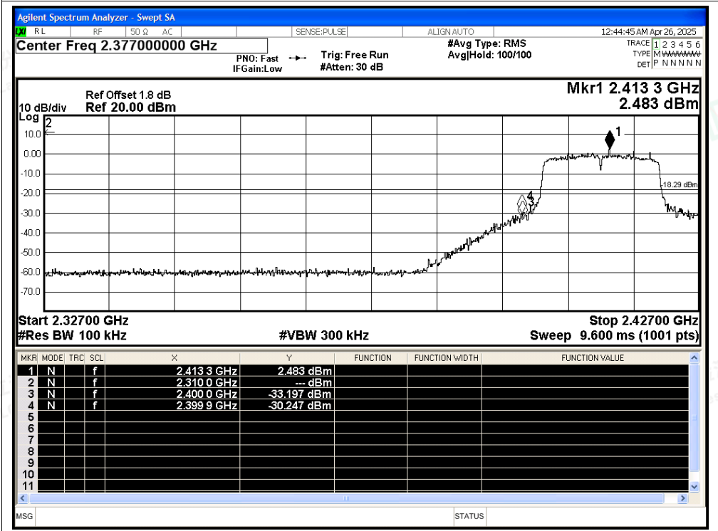
Band Edge NVNT ax20 2412MHz Ant1 Emission
