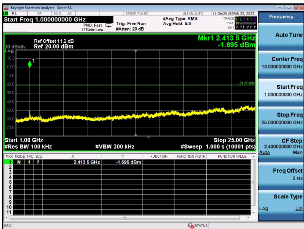
1GHz -25GHz
