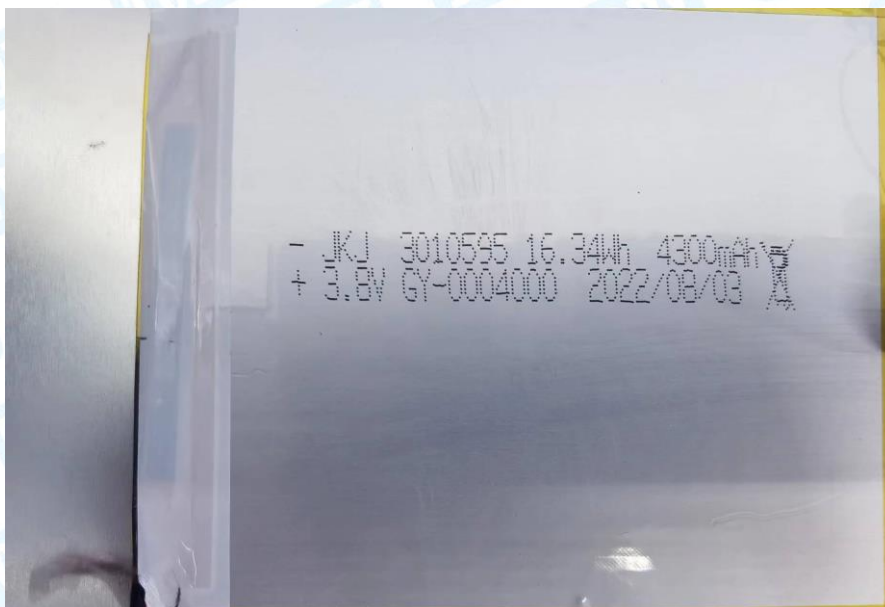
Photo 12 Battery parameters
