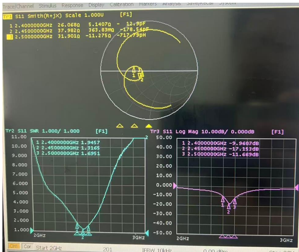
VSWR
