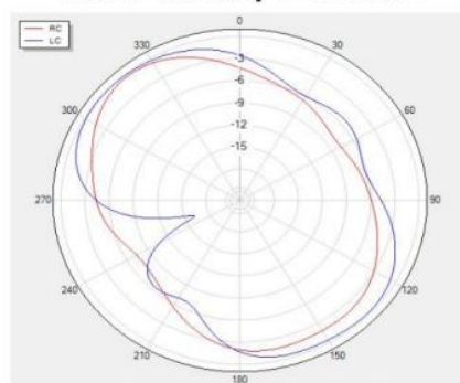
Theta=90 freq=2400MHz
