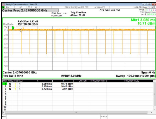
802.11n20
