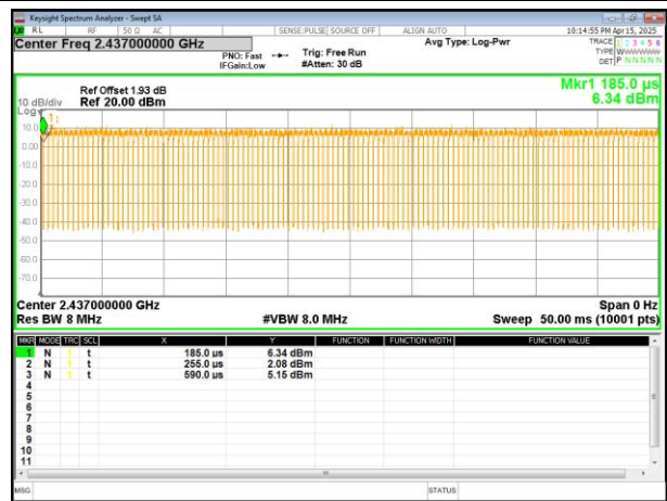
802.11n40
