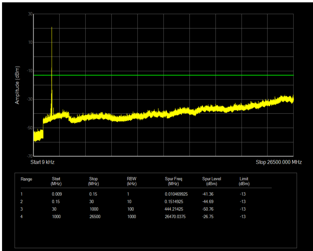
Band2 QPSK Channel=18900 nTones=1@0 Spacing=15kHz
