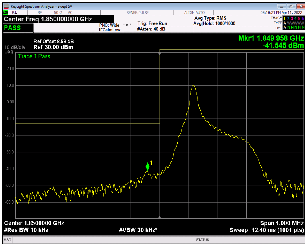
Band2 QPSK Channel=18602 nTones=1@0 Spacing=15kHz
