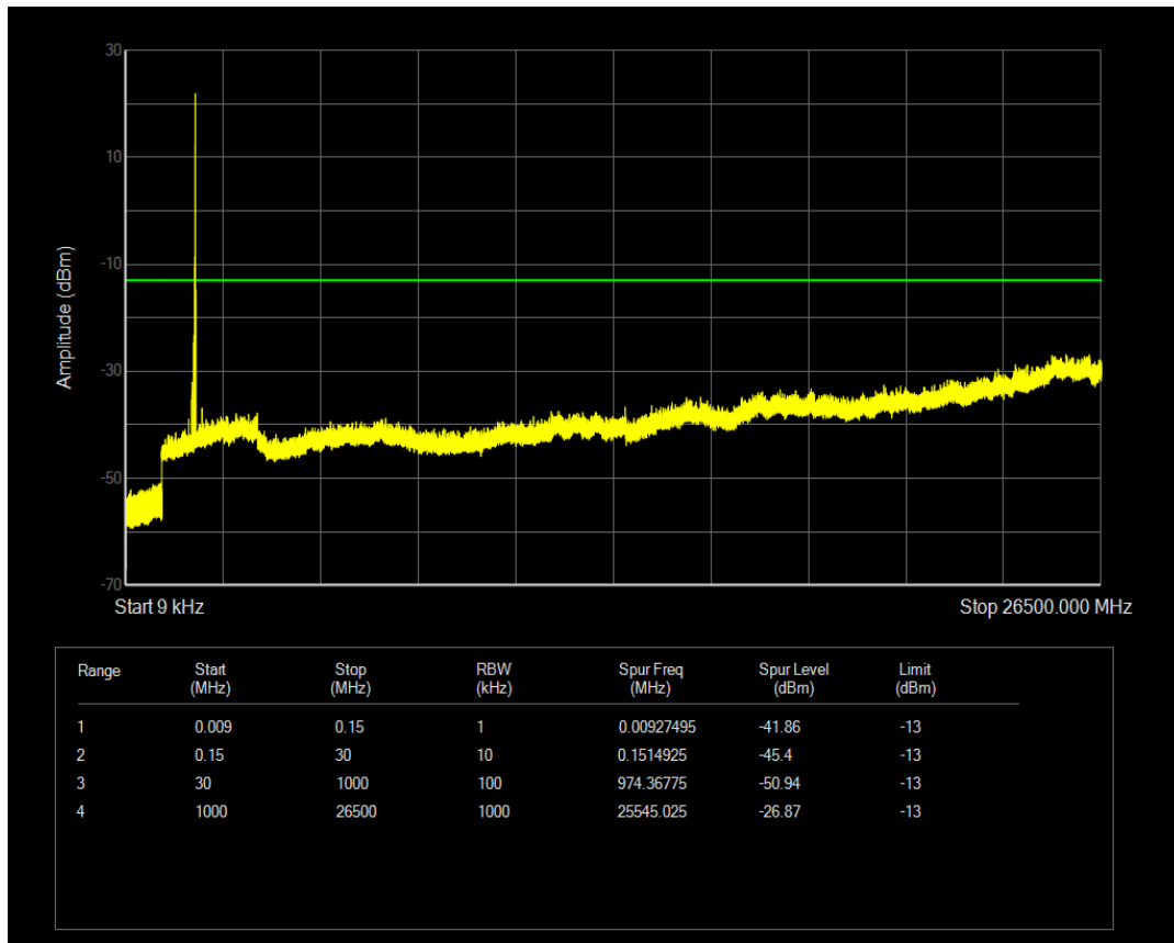
Band2 QPSK Channel=19198 nTones=1@0 Spacing=15kHz
