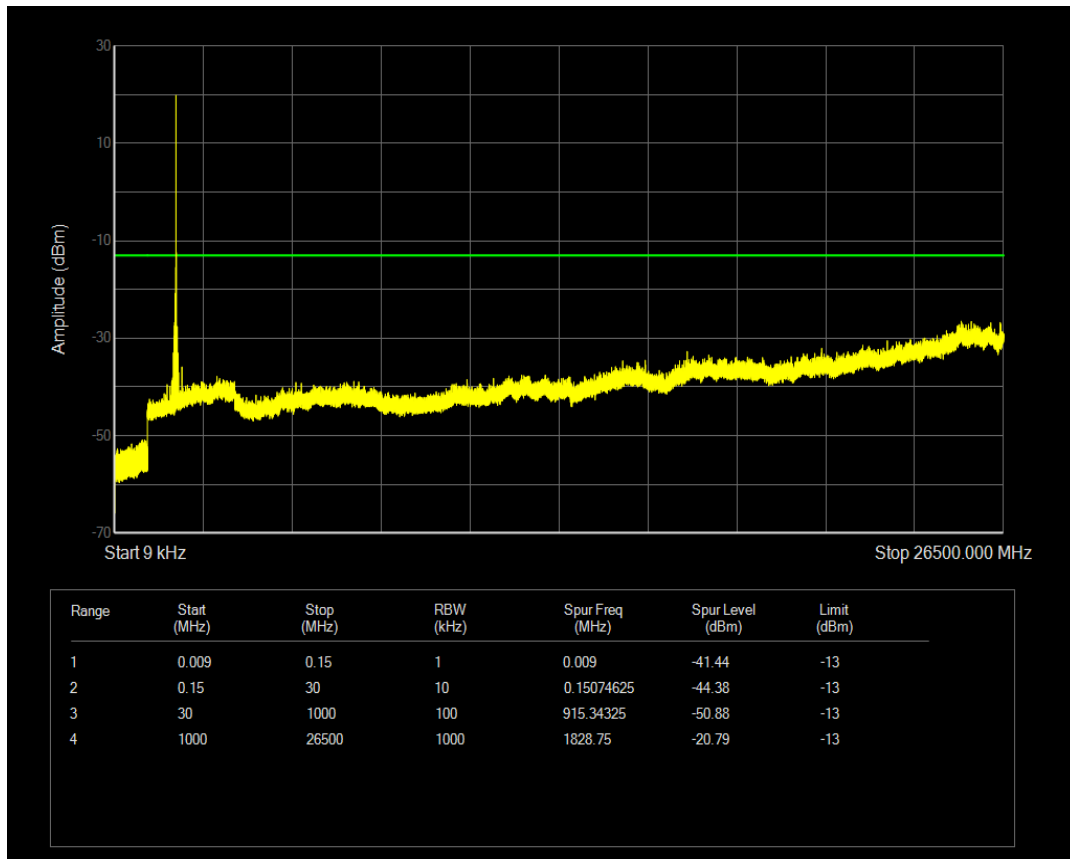
Band2 QPSK Channel=18602 nTones=1@0 Spacing=15kHz
