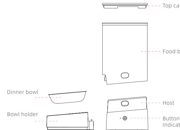
Top cap
