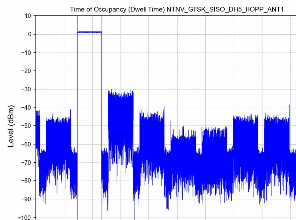
DH5
