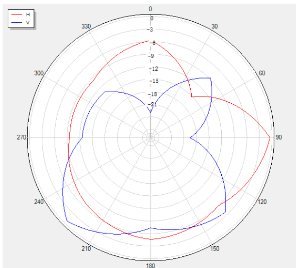
2500 Polar
