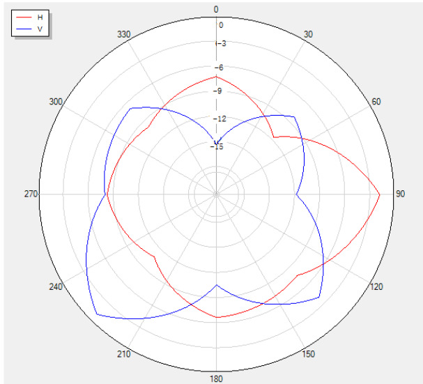
2450 Polar
