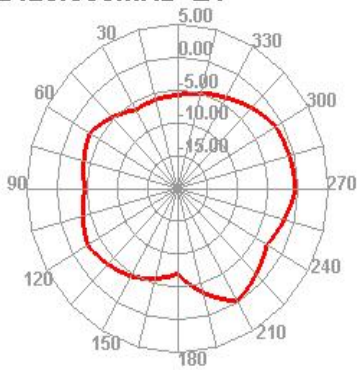
2430.000MHz
