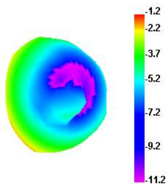
2210.000MHz E1
