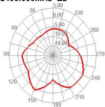
2430.000MHz E2
