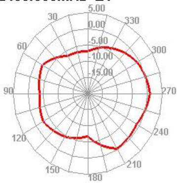
2480.000MHz E1
