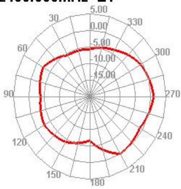
2450.000MHz E1
