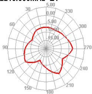
2220.000MHz
