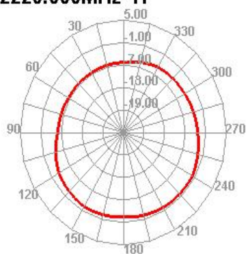
2220.000MHz H
