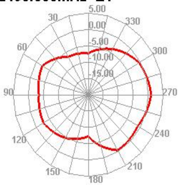
2490.000MHz E1
