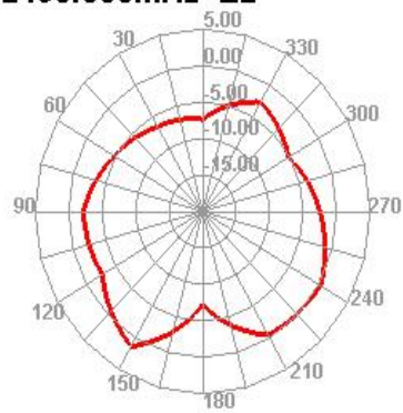
2490.000MHz E2
