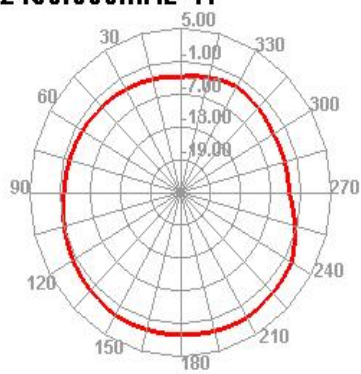
2450.000MHz H
