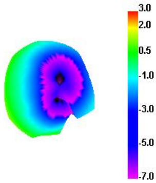
2440.000MHz
