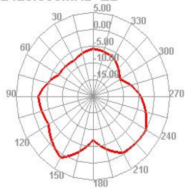
2430.000MHz H
