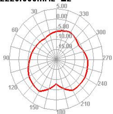
2220.000MHz E2
