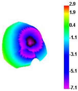
2480.000MHz
