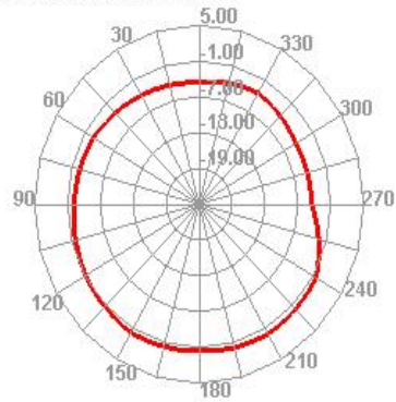
2420.000MHz H
