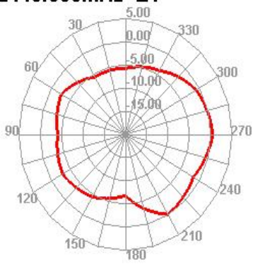
2440.000MHz E1
