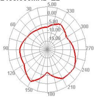
2480.000MHz E2
