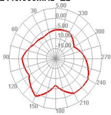
2440.000MHz E2
