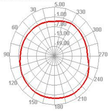
2480.000MHz H
