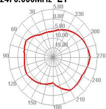
2470.000MHz E1
