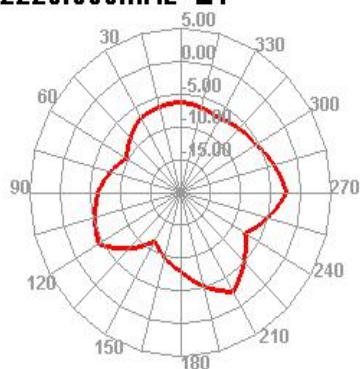
2220.000MHz E1
