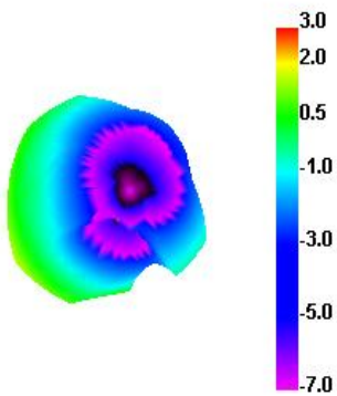
2490.000MHz
