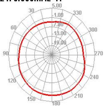
2470.000MHz H
