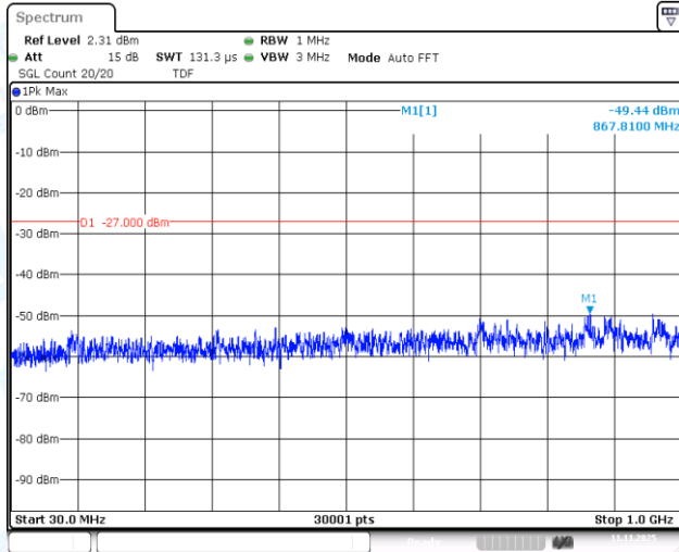
11A-Ant1-5745-30~1000-PASS
