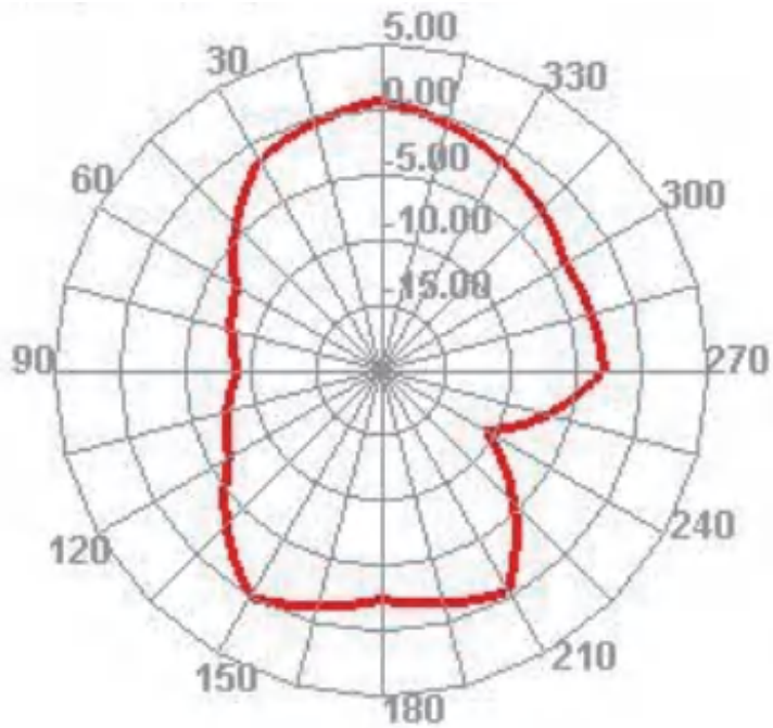
2400MHz
