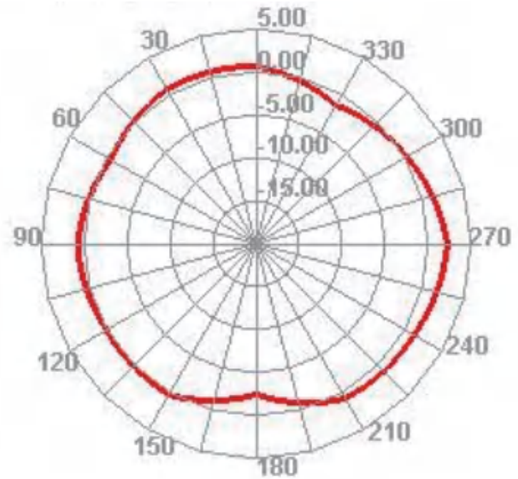
2490MHz
