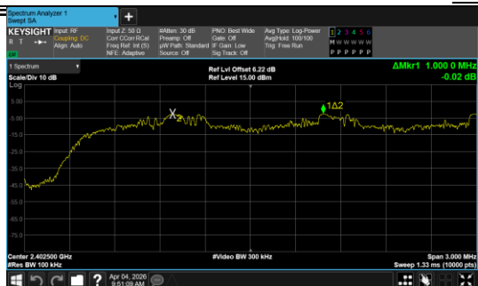
8DPSK
