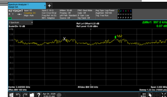
8DPSK
