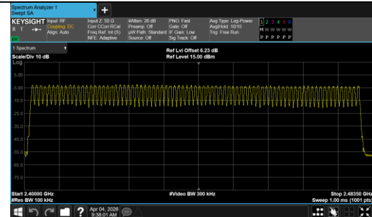
Hopping Plot \pi/4 DQPSK
