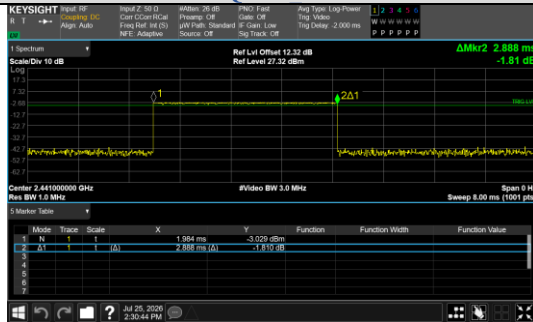
Pulse Width \pi/4 DQPSK 2-DH5
