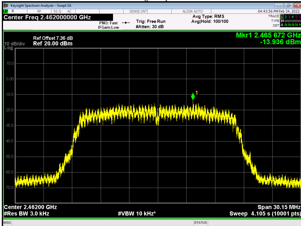
PSD NVNT 802.11g 6Mbps 2462MHz Ant1
