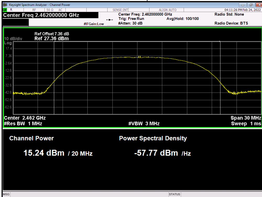
Power NVNT 802.11b 1Mbps 2462MHz Ant1
