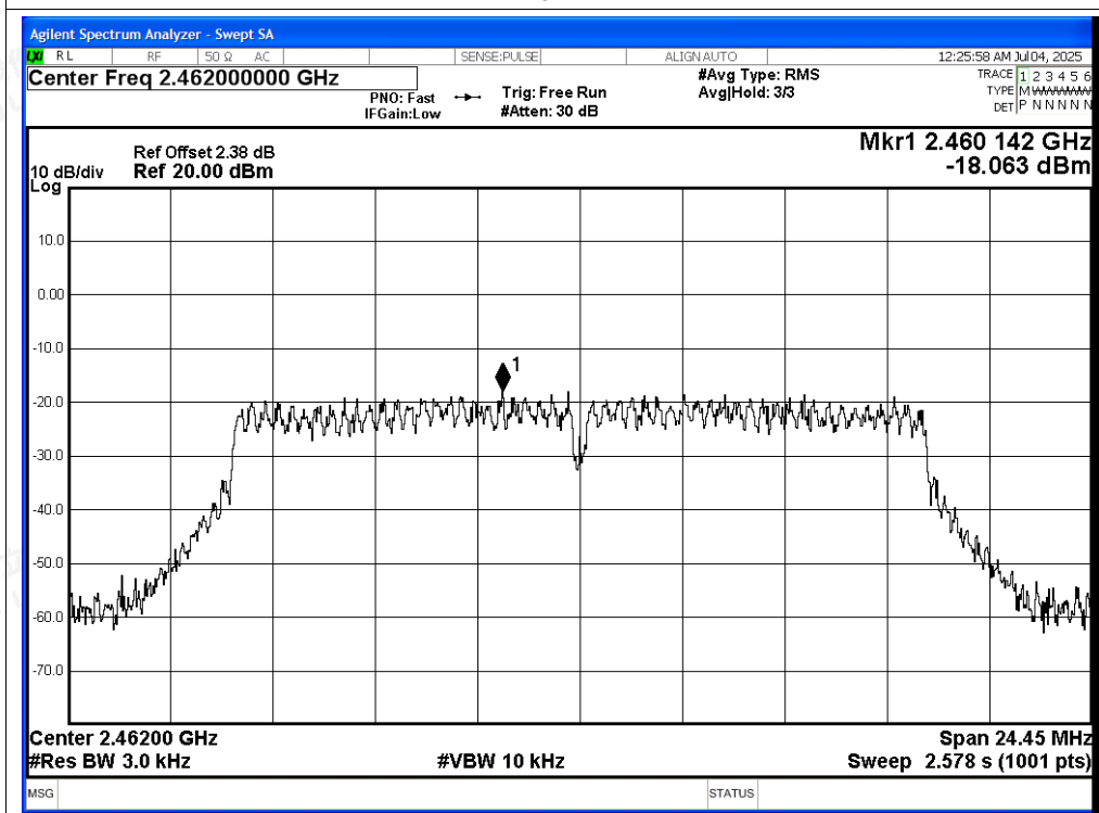
PSD NVNT g 2462MHz Ant1
