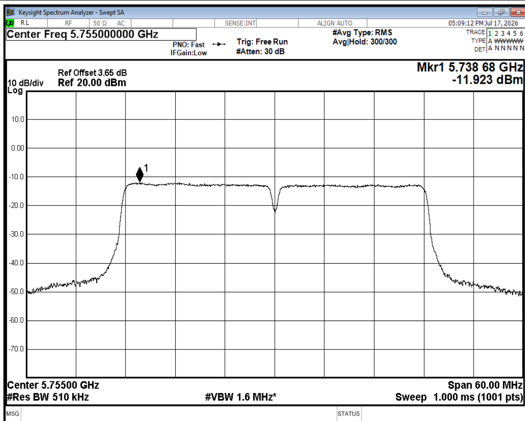
PSD NVNT n40 5755MHz Ant1
