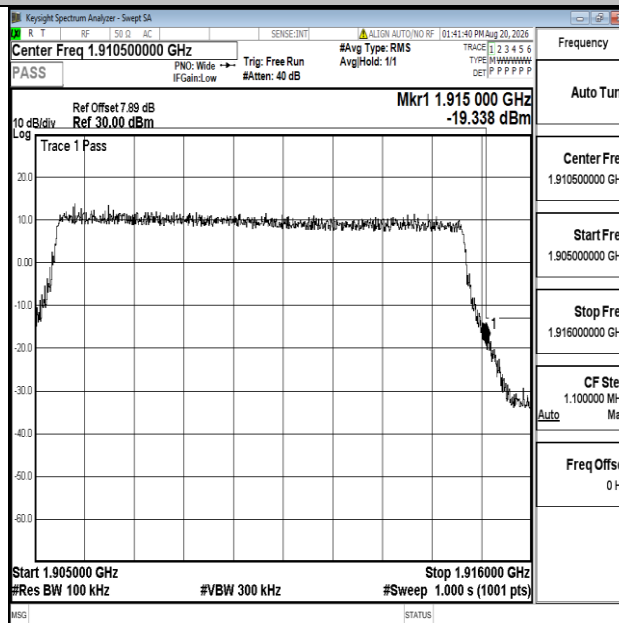
Band25-10MHz-QPSK-26640-50RB#0-PASS
