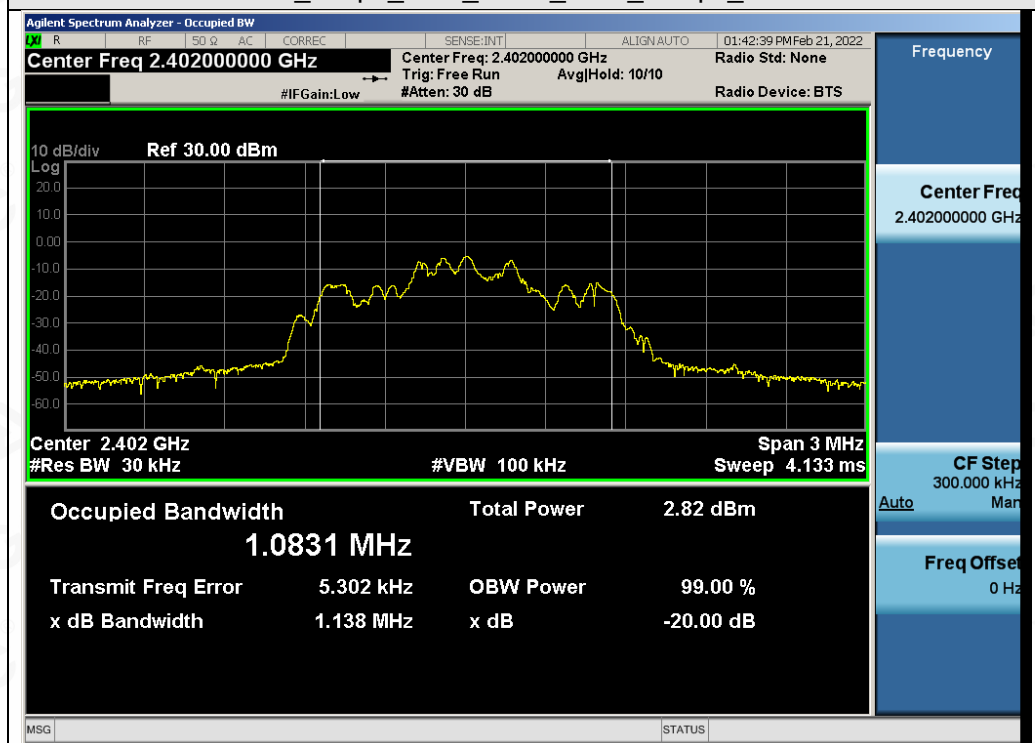
Test_Graph_EDR_ANT1_2402_3Mbps_OBW
