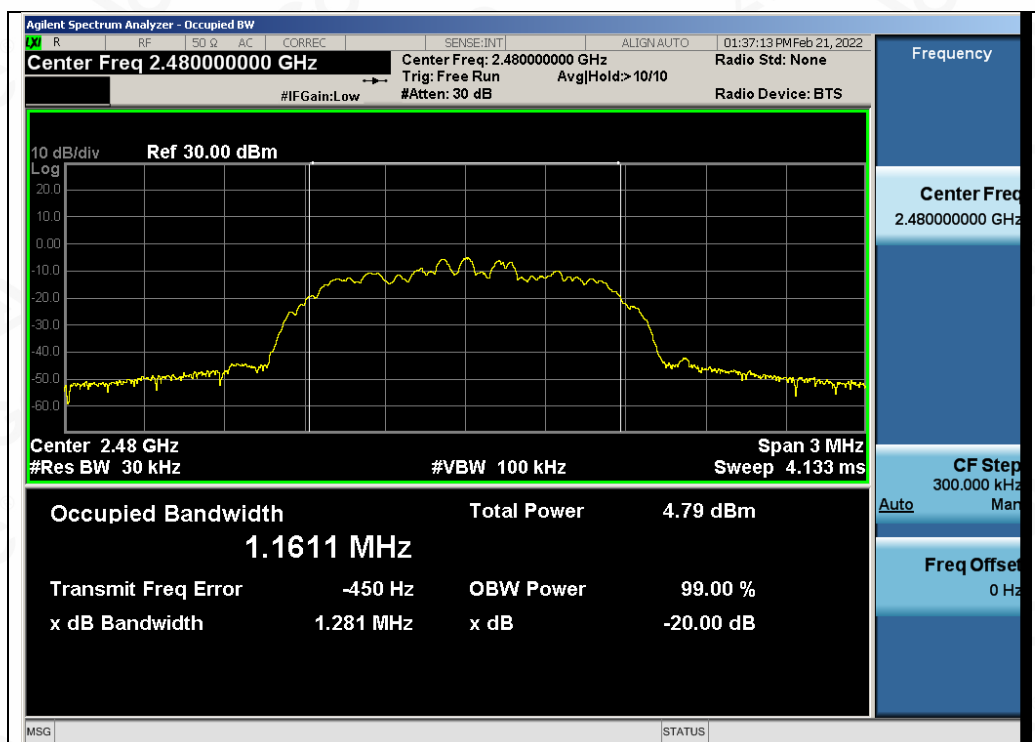
Test_Graph_EDR_ANT1_2480_2Mbps_OBW
