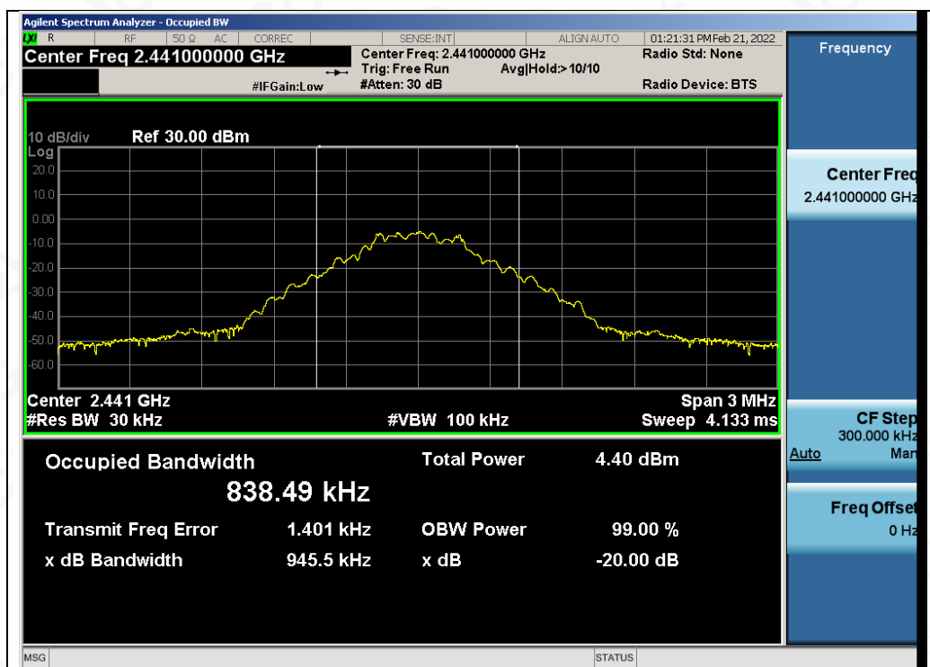
Test_Graph_BR_ANT1_2441_1Mbps_OBW
