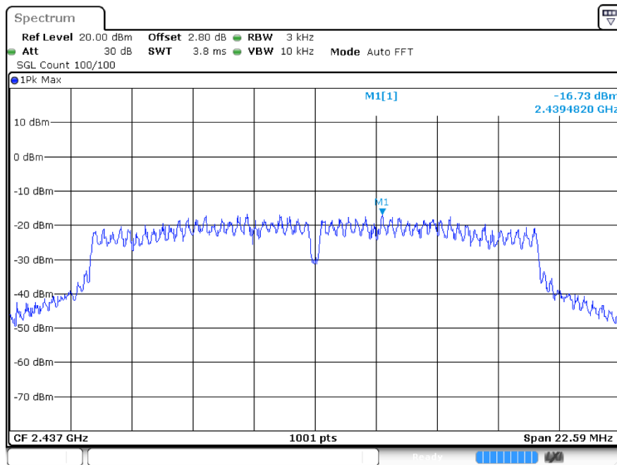
PSD g 2437MHz Ant1
