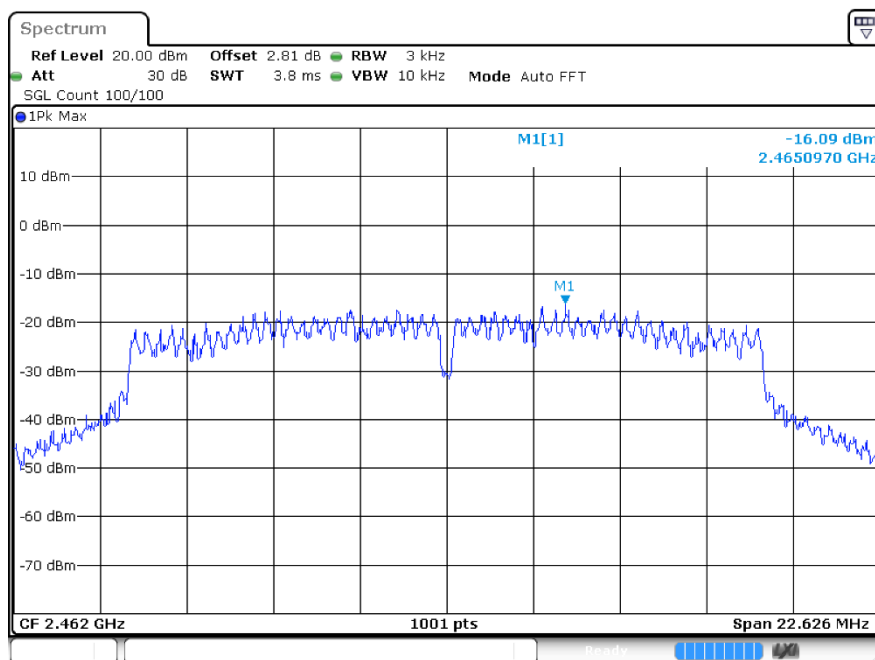
PSD g 2462MHz Ant1
