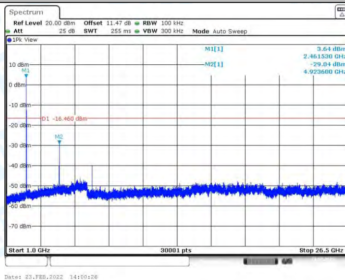
11B_Ant1_2462_1000~26500
