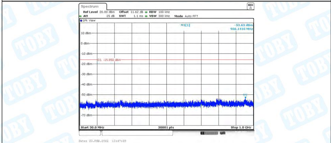
11B_Ant1_2412_30~1000
