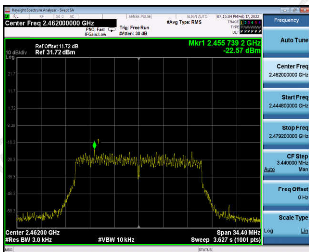
CH11
