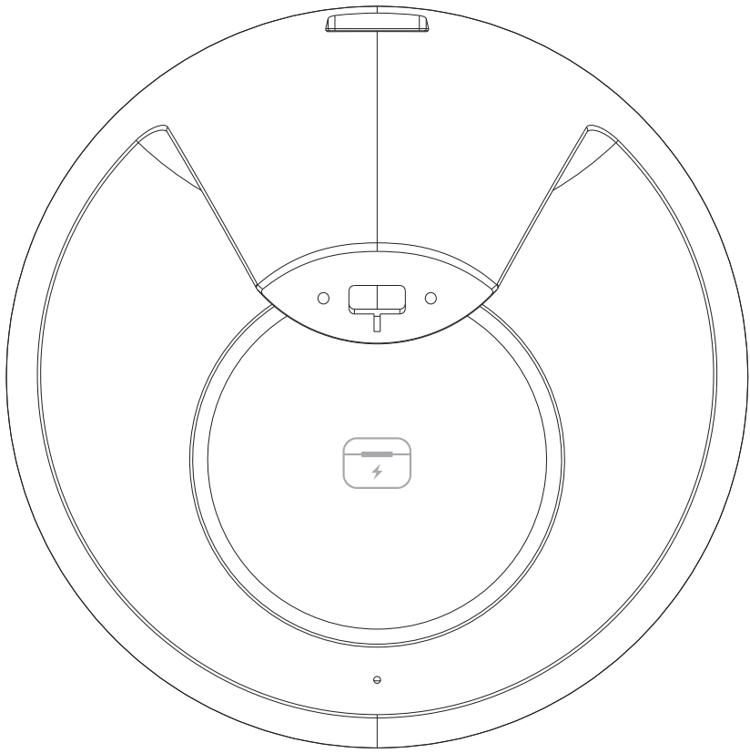
耳机充电图标丝印位置
