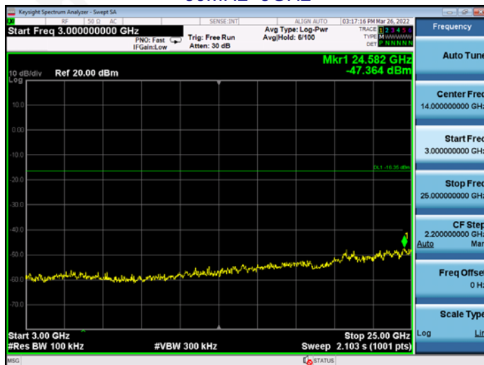
3GHz~25GHz
