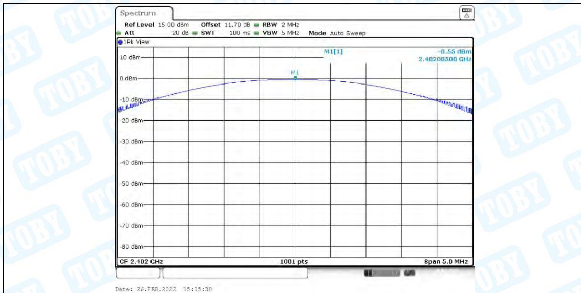
DH5_Ant1_2402
