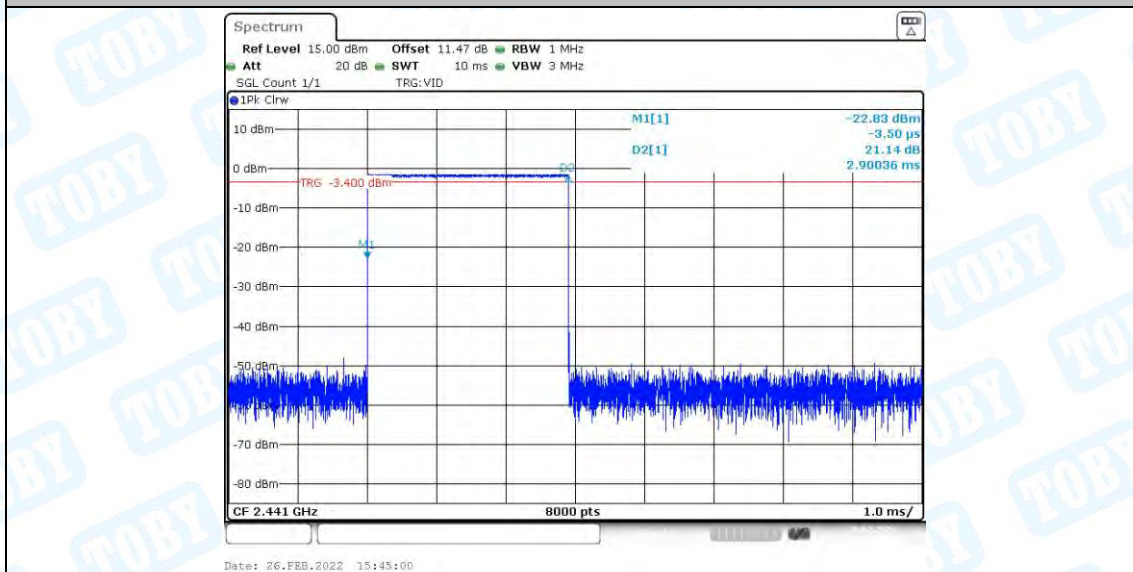
DH5_Ant1_Hop
