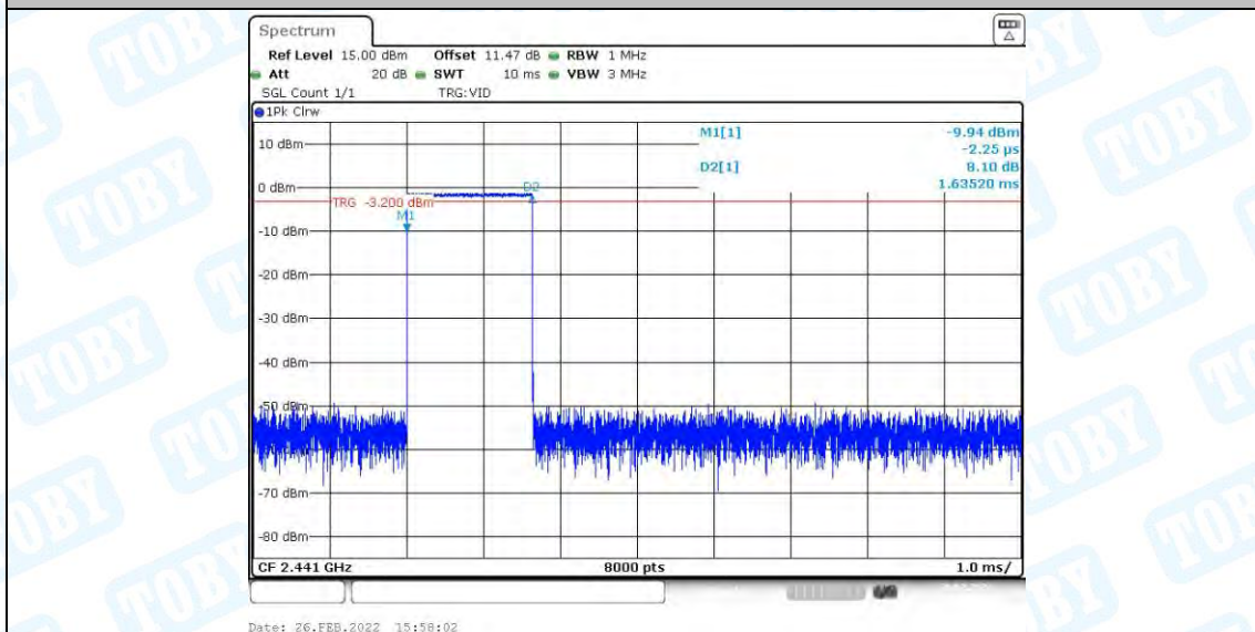
DH3_Ant1_Hop
