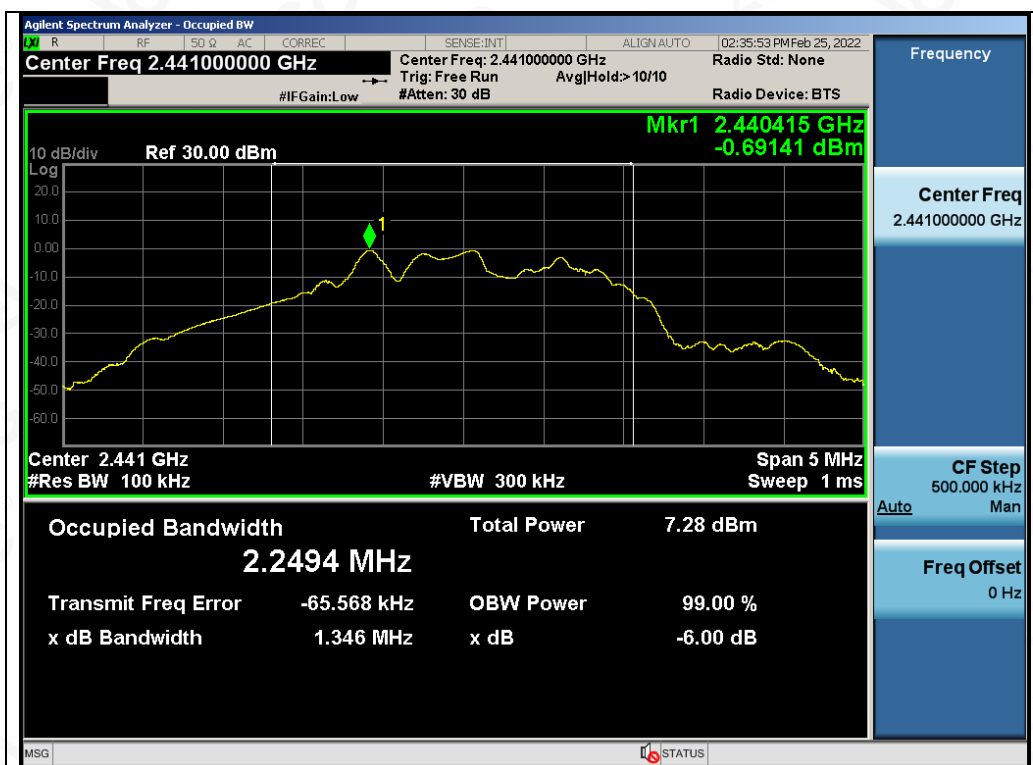
Test_Graph_GFSK_ANT1_2441_DTSBW
