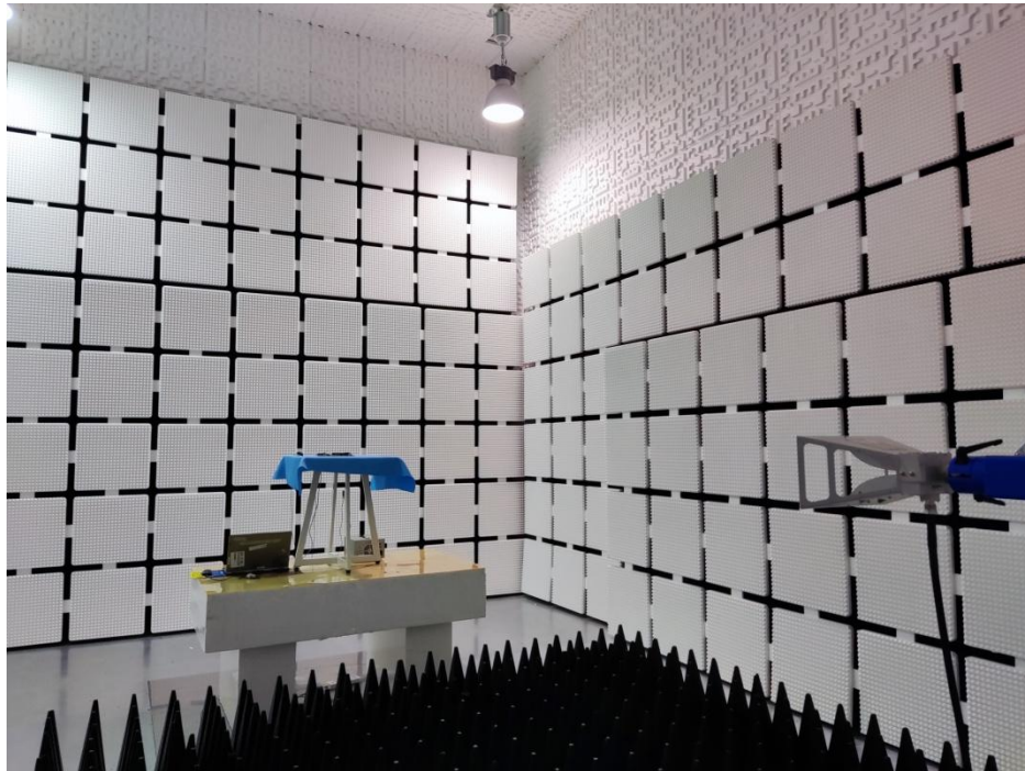
RSE 1GHz-18GHz
