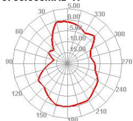
5750.000MHz E2
