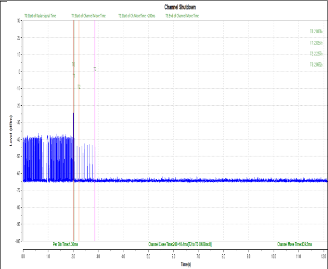
11AX80SISO-5530-Type0-PASS
