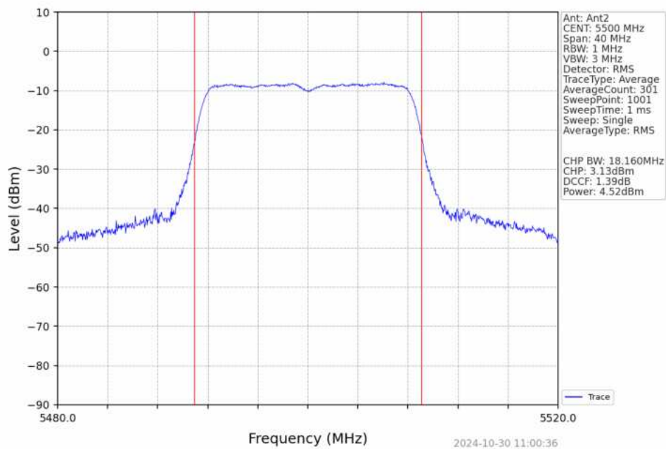
802.11a_LCH_5500MHz_Ant2_NTNV
